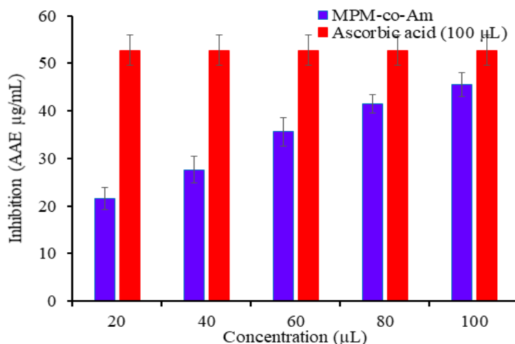
Fig. 1. DPPH test
